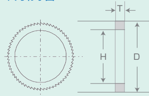
尺寸标示图
